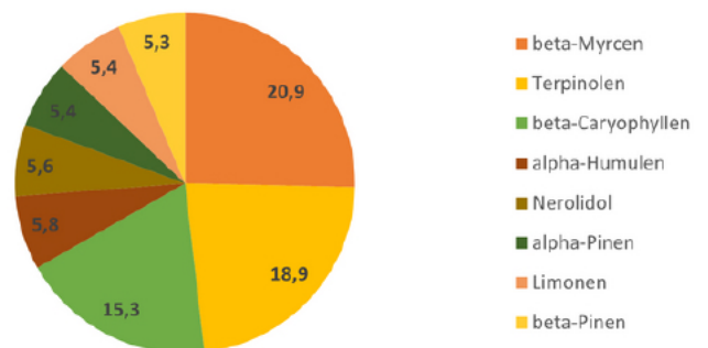
Terpendiagramm
